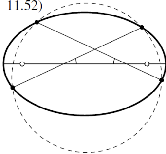
11.3.12)
