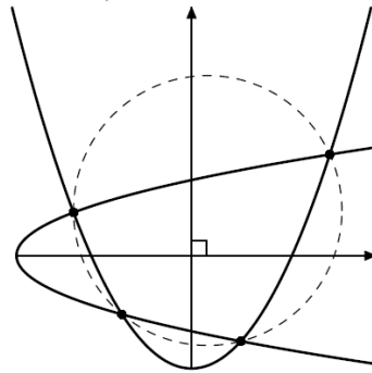
11.3.13)
