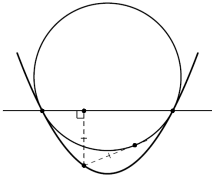
11.1.21)
